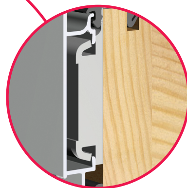
DIMEZZAMENTO DEL TEMPO DI INSTALLAZIONE impiegando apposite clips con passo 400 mm
