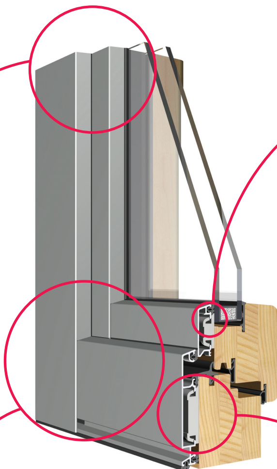
CLIPS con funzione di fermavetro in sicurezza
